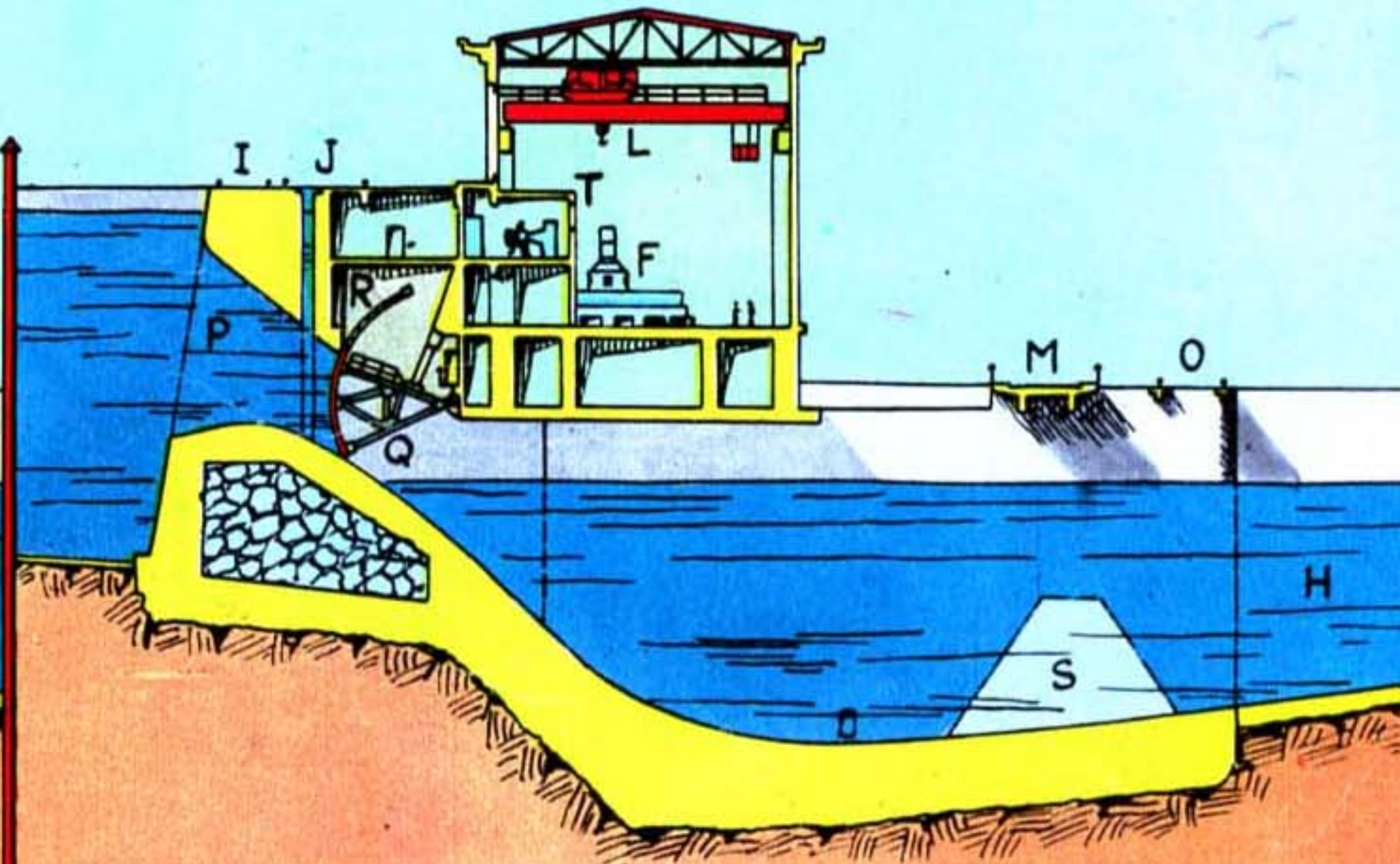
COUPE DANS L'AXE D'UN DÉCHARGEUR
