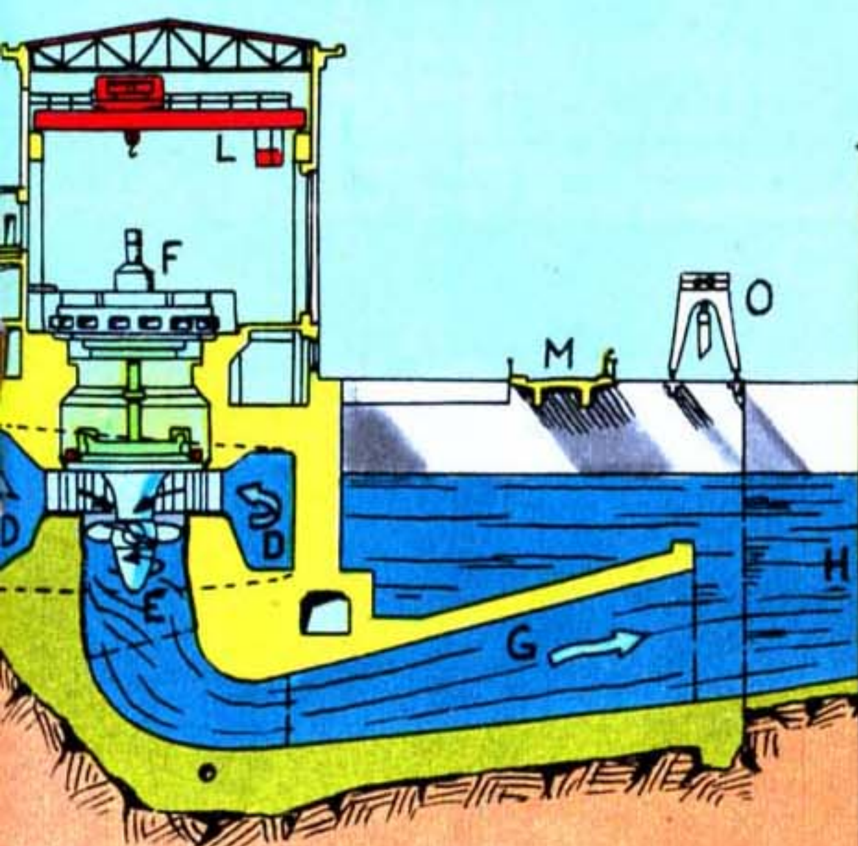
COUPE D'UN GROUPE TURBO-ALTERNATEUR
