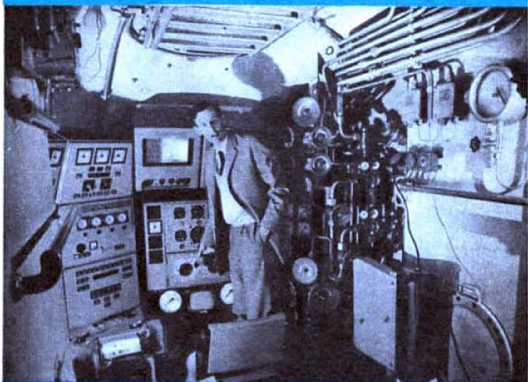
L'inventeur, J. Piccard, montre le tableau de bord du sous-marin.
