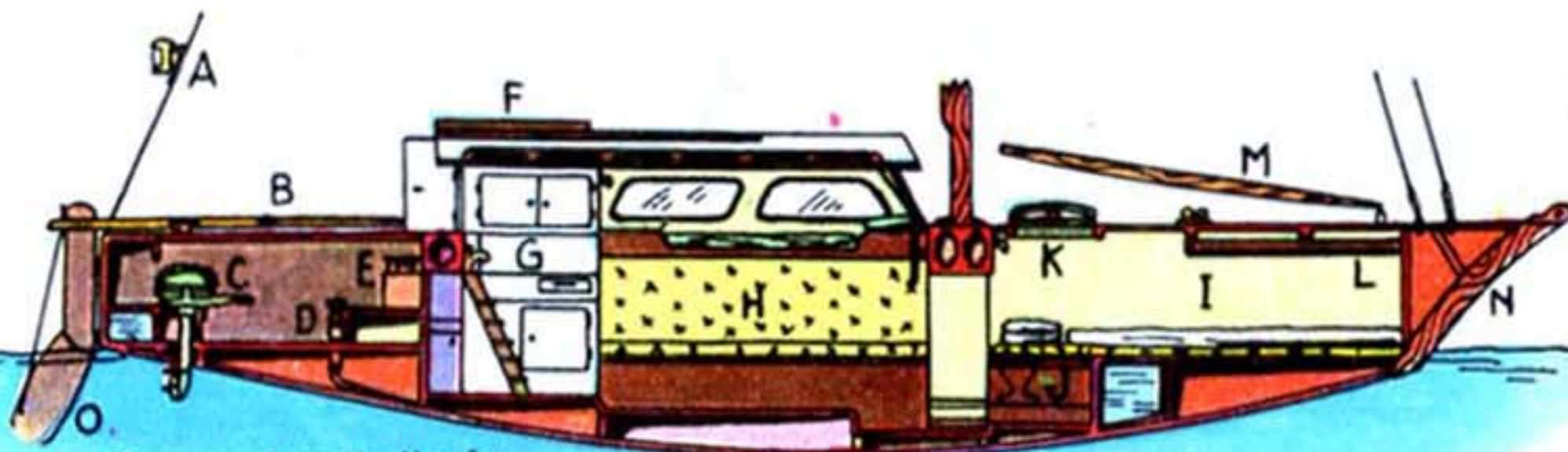
Coupe longitudinale de la coque centrale.
